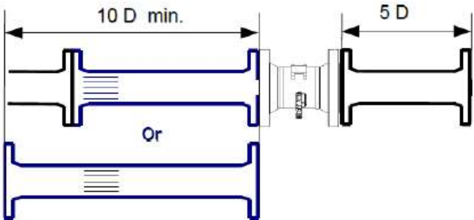
DISPOSIÇÃO DO CONDICIONADOR DE FLUXO
